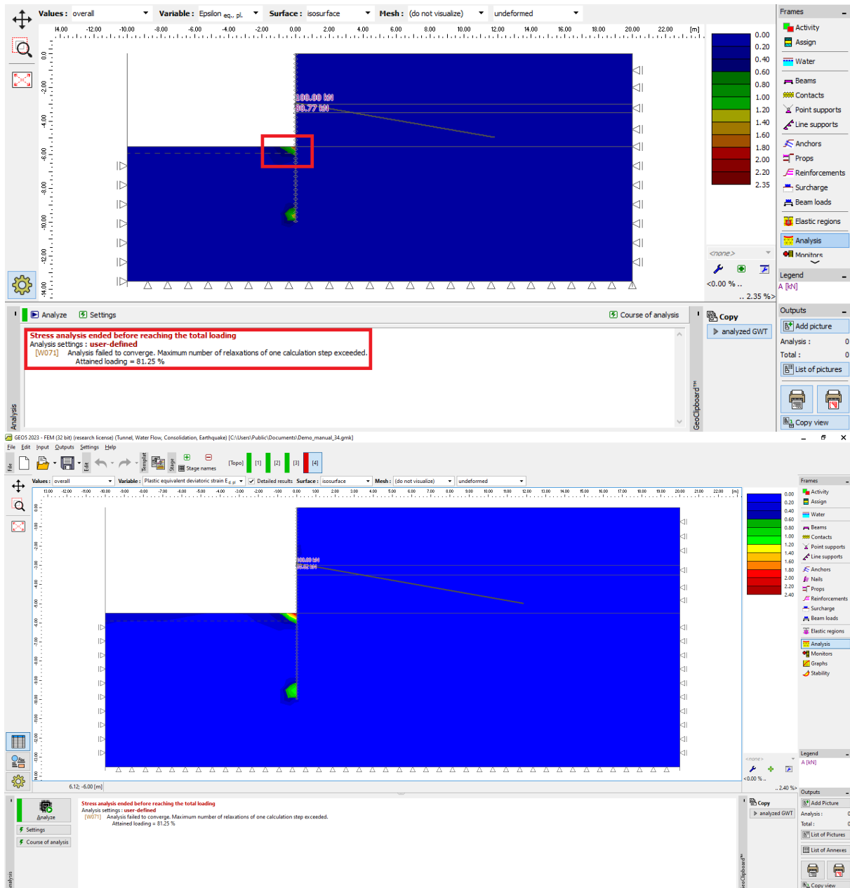
Equilíbrio para a carga total não alcançado na 4ª etapa – sem redistribuição de deformações plásticas, divergência na análise
