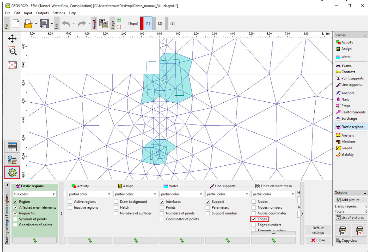
Configuração da malha de elementos finitos
