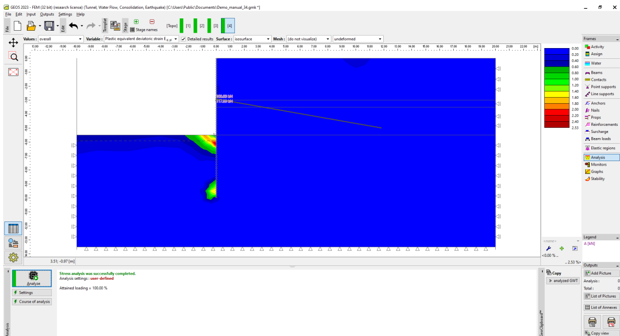
Equilíbrio alcançado para 4ª etapa utilizando uma região elástica
