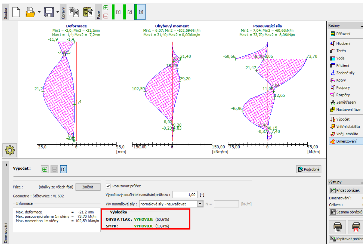
Rám „Dimenzování“ – fáze budování 3 (využití ocelové štětovnice typu VL 602)
