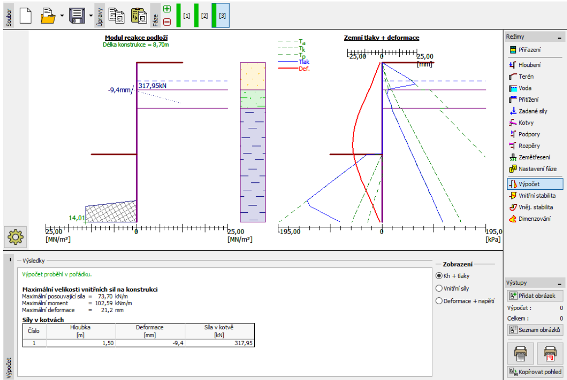
Rám „Výpočet“ – Fáze budování 3 (Kh + tlaky)
