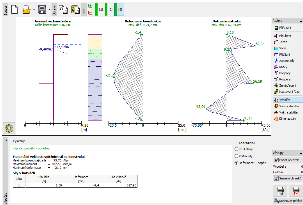
Rám „Výpočet“ – Fáze budování 3 (deformace + napětí)
