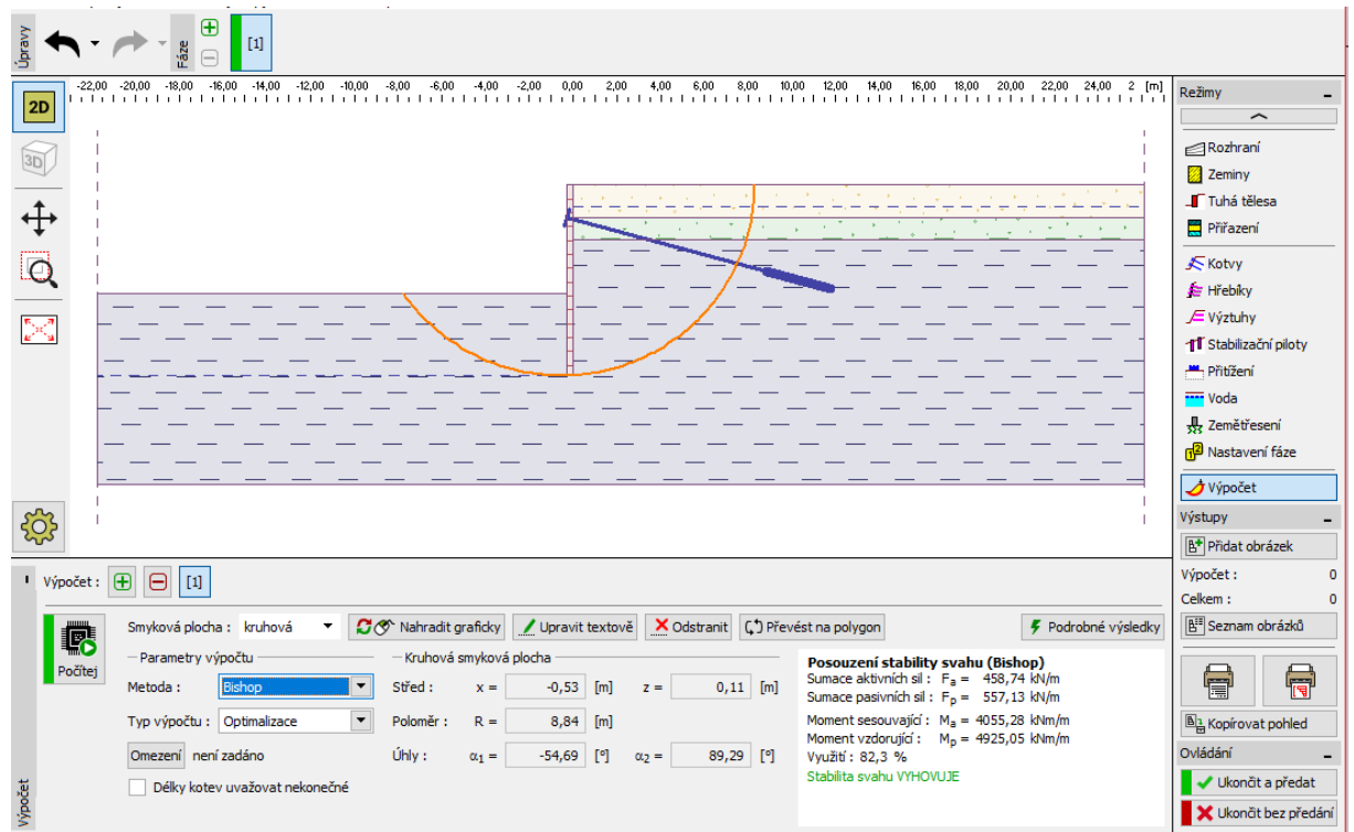
Rám „Vnější stabilita“
