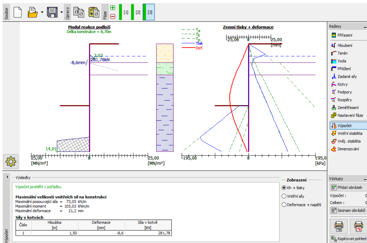
Rám „Výpočet“ – po změně délky kotvy
