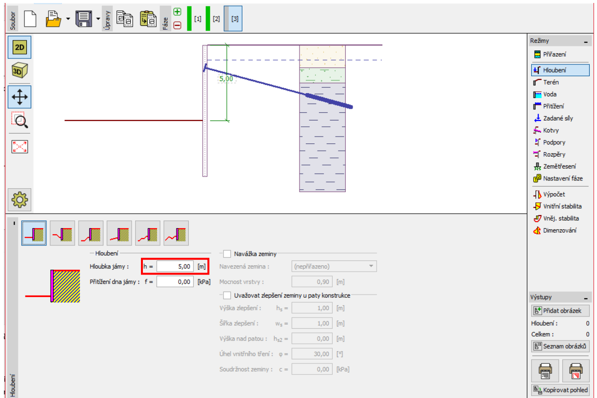
Rám „Hloubení“ – fáze budování 3
