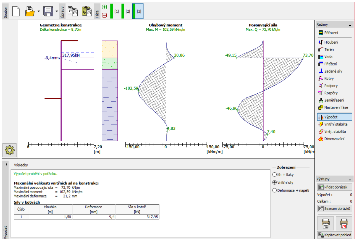
Rám „Výpočet“ – Fáze budování 3 (vnitřní síly)
