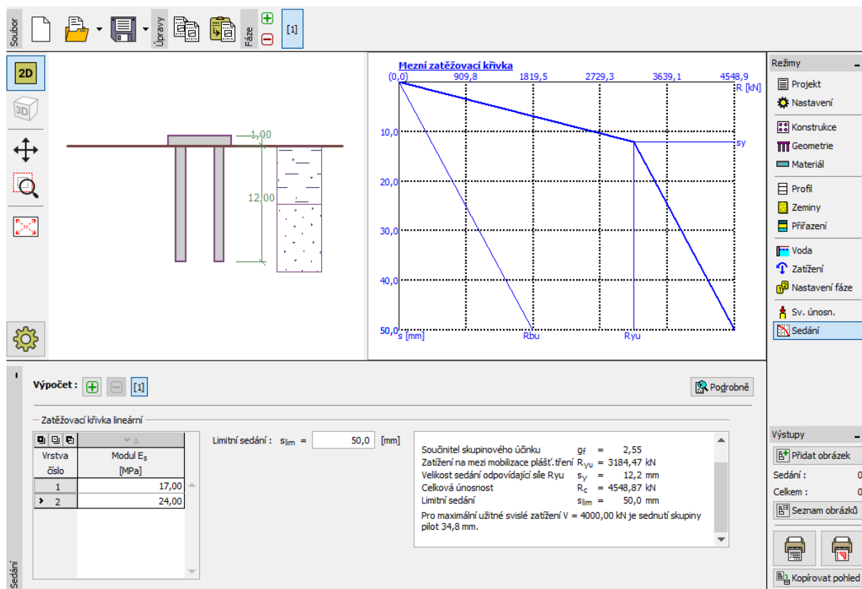
Rám „Sedání“ – metoda NAVFAC DM 7.2
