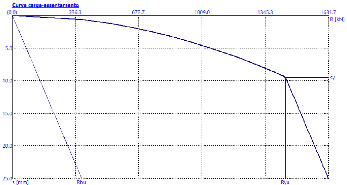
“Janela “Assentamento” – curva de carregamento não linear (segundo Masopust)
