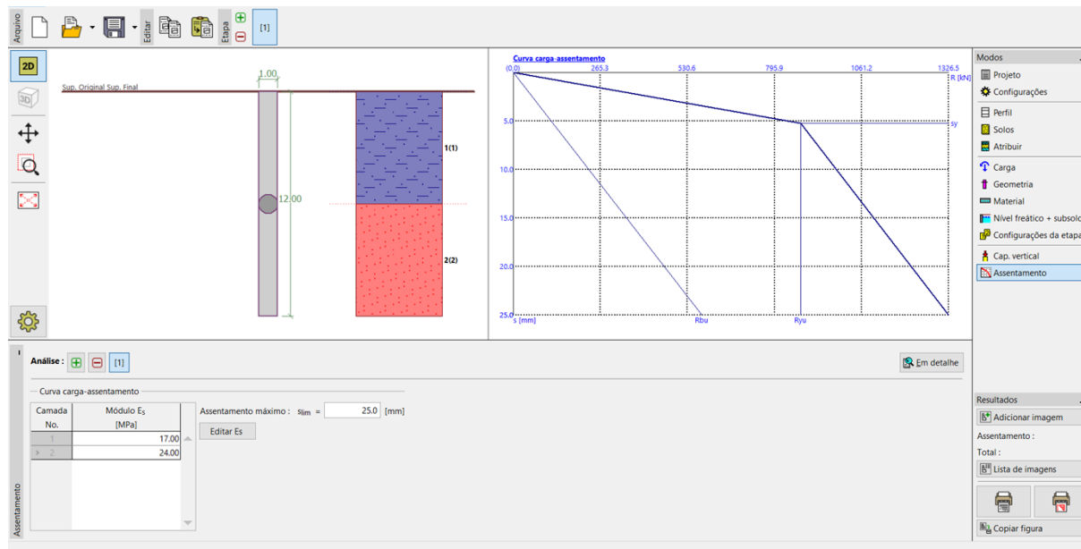
Janela “Assentamento” – curva de carregamento linear (segundo Poulos)
