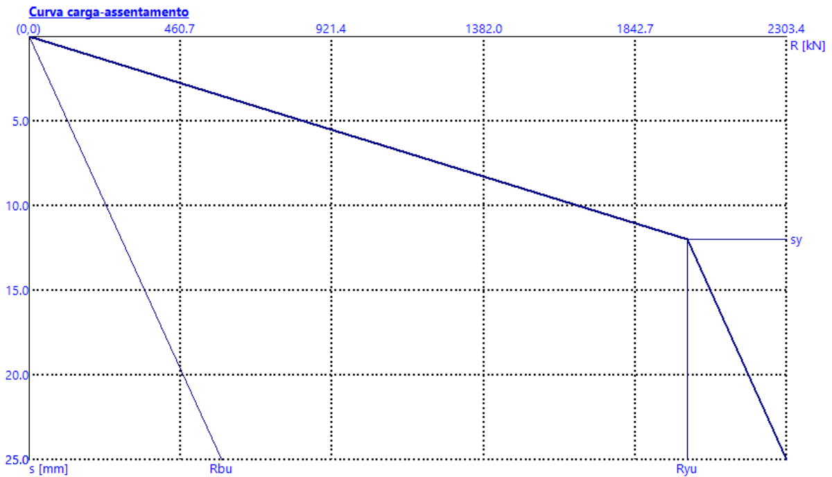
Janela "Assentamento" – curva de carregamento linear (segundo Poulos) para o método da tensão efetiva
