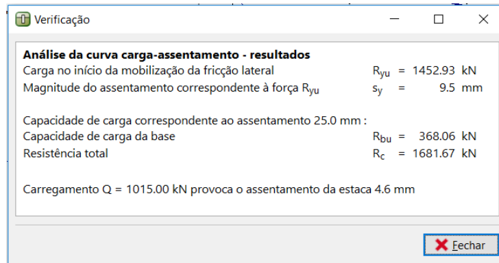
Resultados de assentamento – curva não linear
