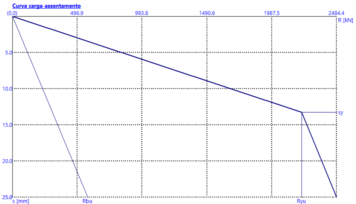
Janela "Assentamento" – curva de carregamento linear (segundo Poulos) para o método CSN 73 1002
