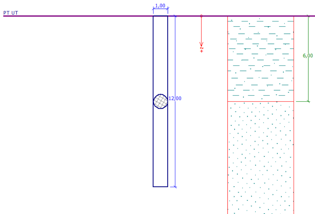
Esboço do problema – estaca isolada
