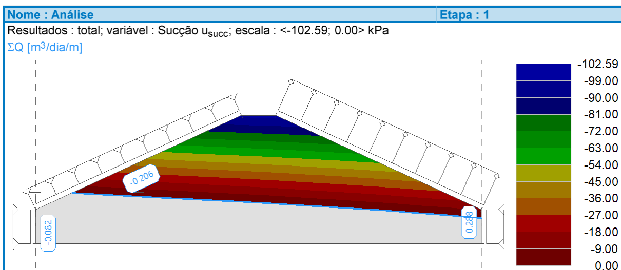
Distribuição da pressão nos poros e sucção (pressão nos poros acima do nível freático) na etapa 1 – estado constante inicial
