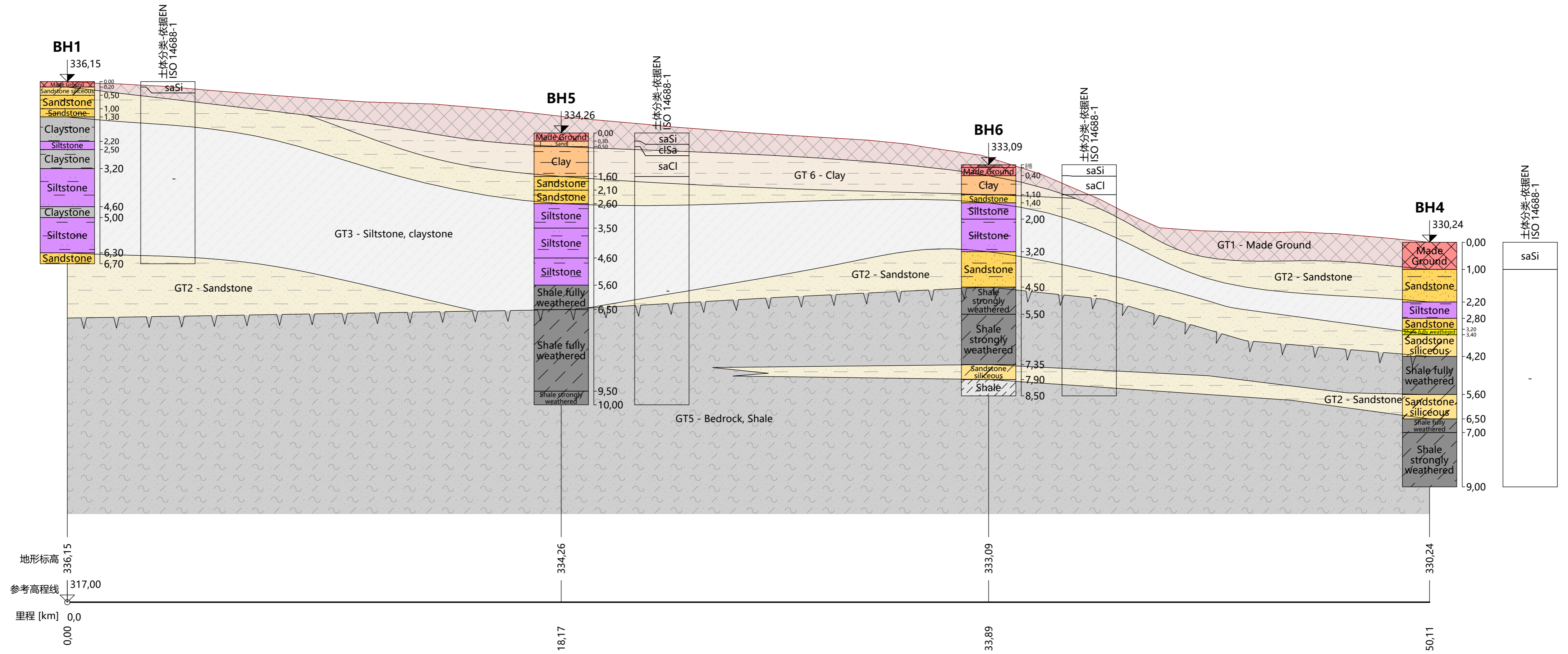
地质剖面 比例尺 1:100/100
