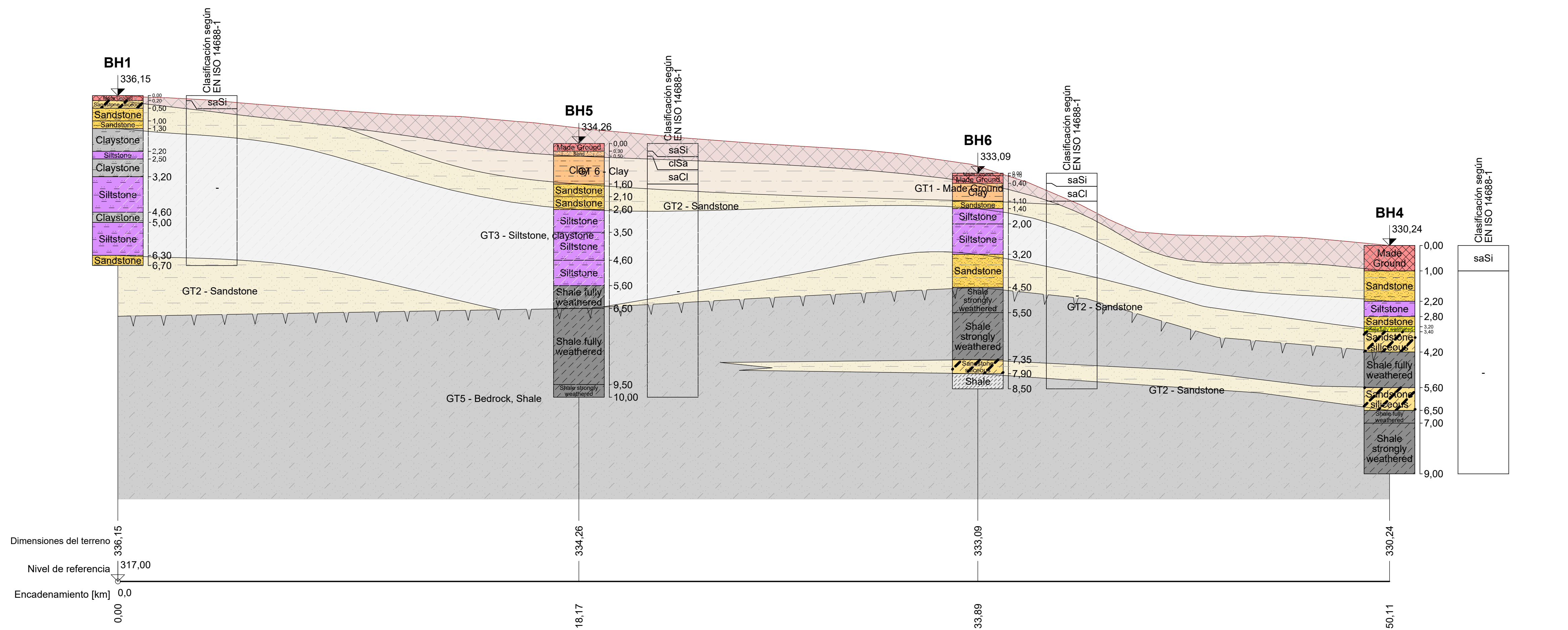
SECCION GEOLOGICA S 1:100/100
