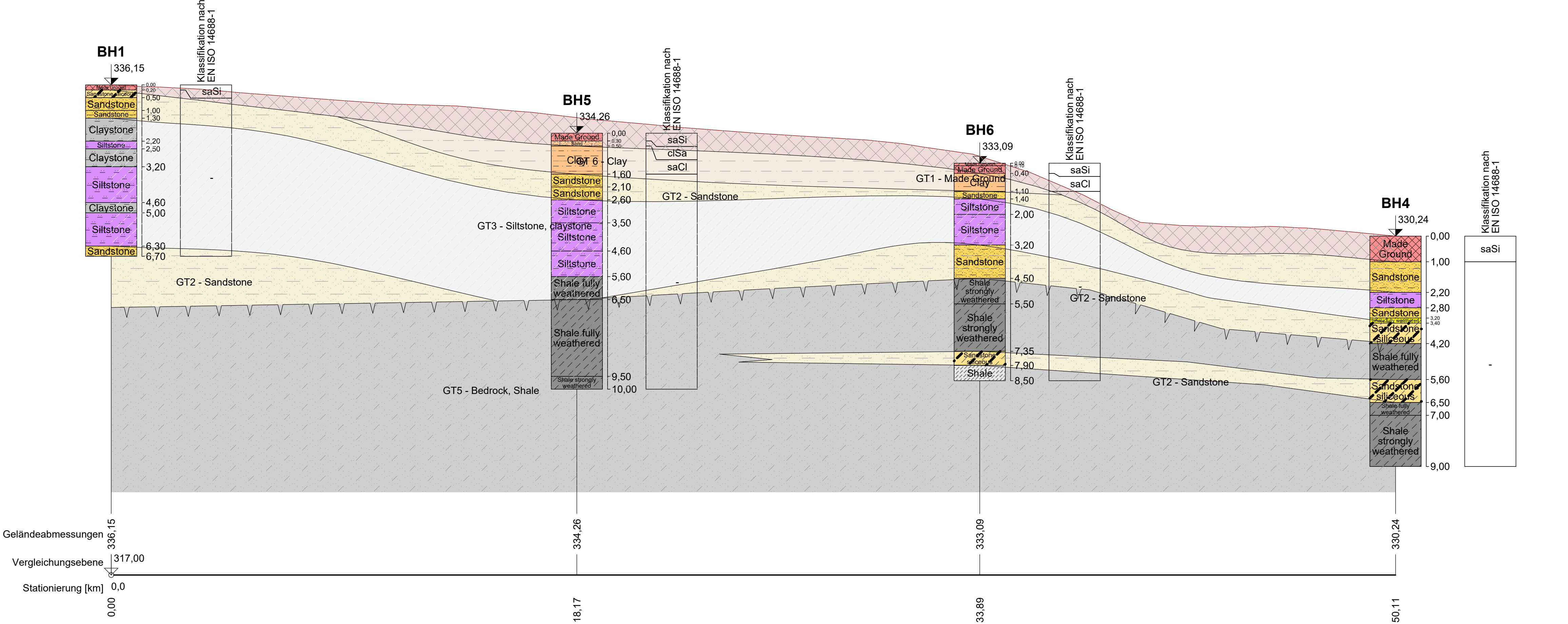
IG Schnitt M 1:100/100
